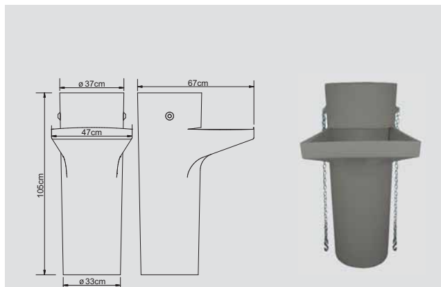
Duto de resíduos intermediário
